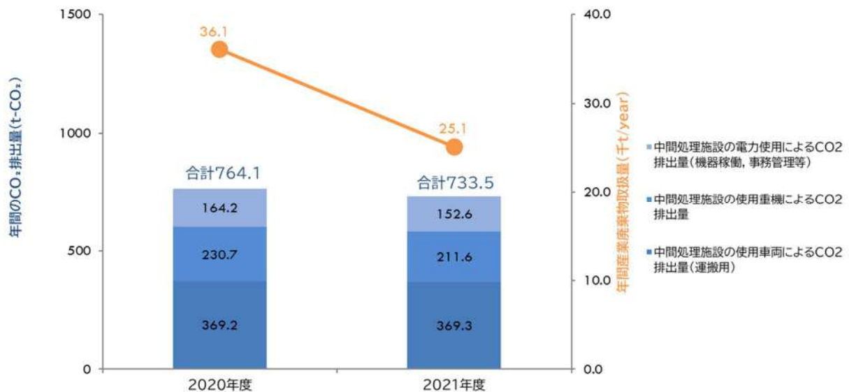
年間CO 2 排出量内訳 2021年度
